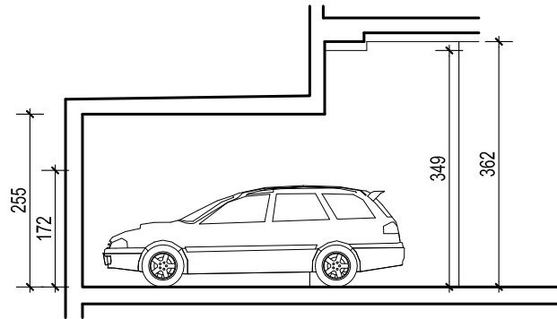
PRESJEK
