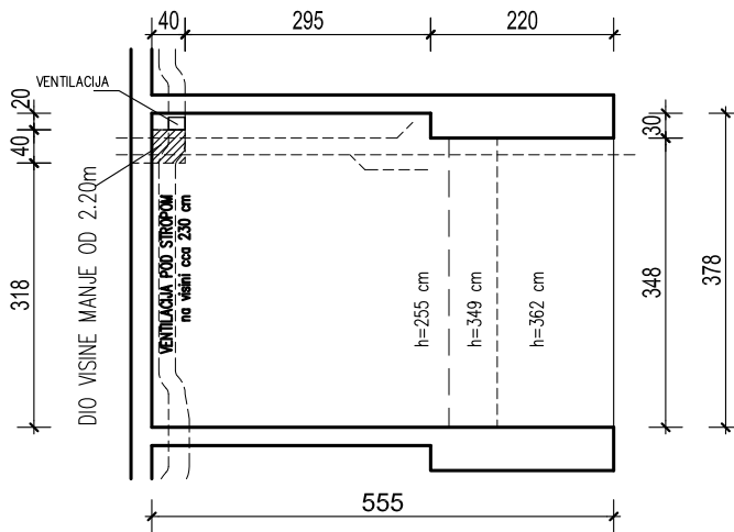
TLOCRT
