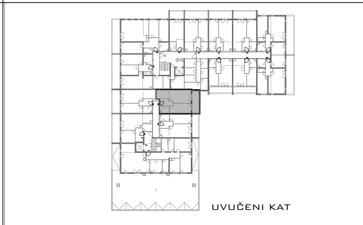
TLOCRT STANA
