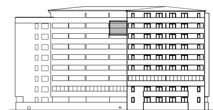
ISTOČNO PROČELJE
