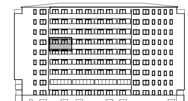
SJEVERNO PROČELJE
