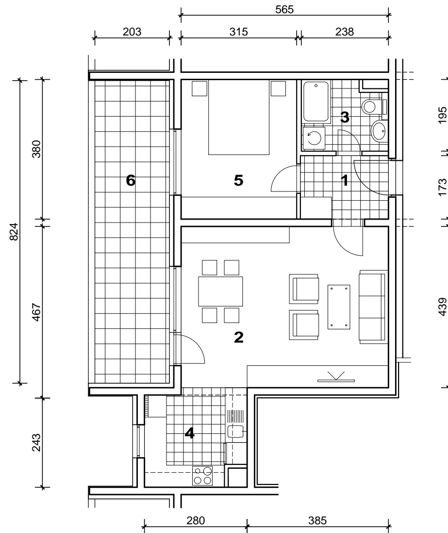
MJ 1:100
