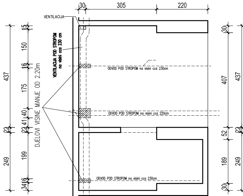
TLOCRT
