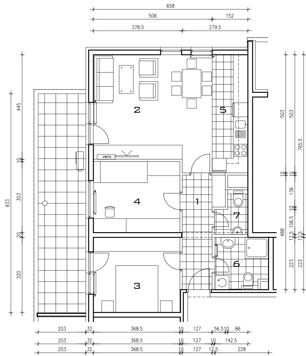
TLOCRT STANA - MJERILO 1:100
